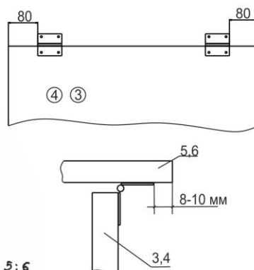
Рис.5 Крепление картонных петель.
