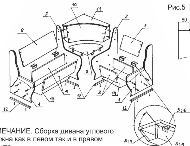
Рис.4 Схема сборки углового дивана
