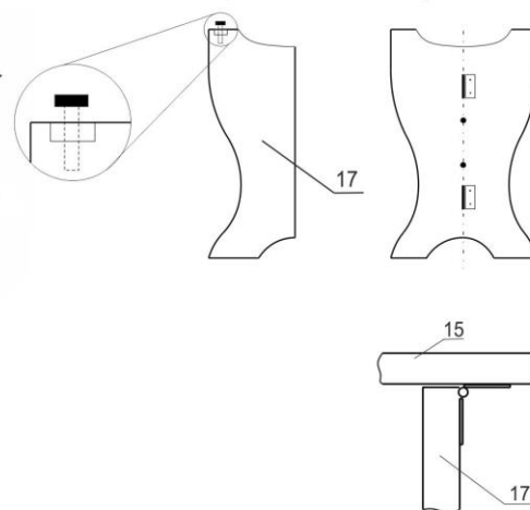
Рис.6 Крепление полуноги.
