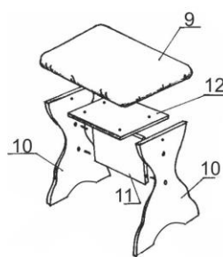
Рис.3 Схема сборки табурета
