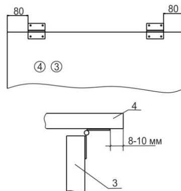
Рис.5 Крепление карточных петель.
