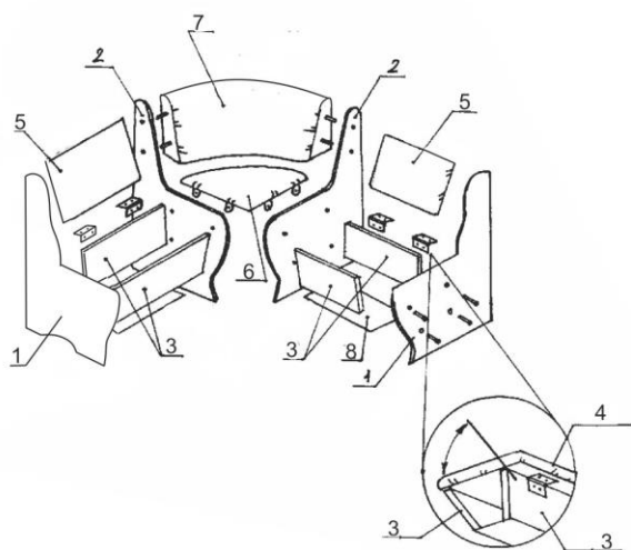
Рис.4 Схема сборки углового дивана
