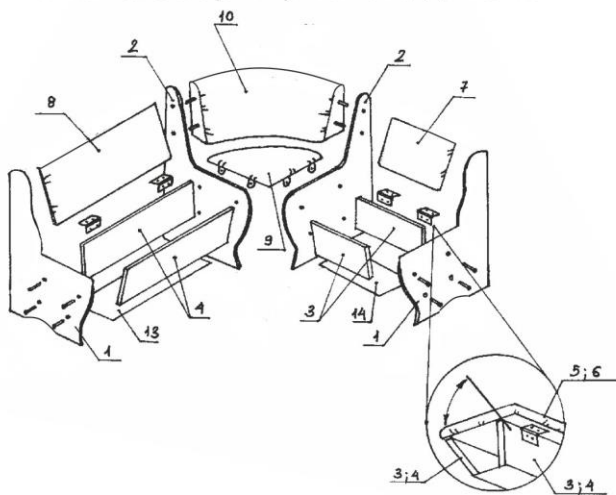
Рис.4 Схема сборки углового дивана
