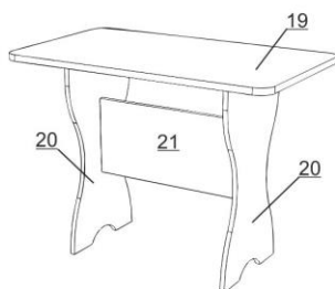
Рис.3 Схема сборки стола.
