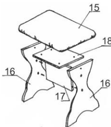
Рис.2 Схема сборки табурета
