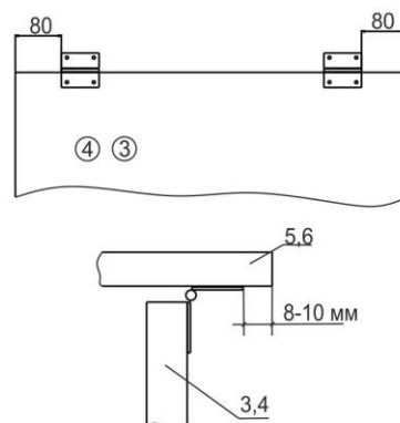
Рис.4 Крепление картонных петель.
