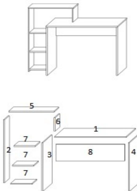
Схема сборки.
