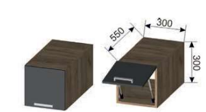
Корпус ШАН 300 (ШхВхГ) 300x300x550 мм Фасад ШАН 300 (ШхВхГ) 296x296x16 мм (1 шт.)
