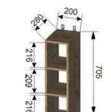
Корпус ШВО 200 (ШхВхГ) 200x705x280 мм
