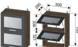
Корпус ШВГ 500 (ШхВхГ) 500x705x280 мм Фасад ШВГГС 500 (ШхВхГ) 496x350x16 мм (2 шт.)
