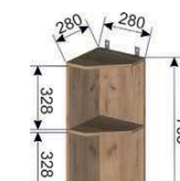
Корпус ШВПГ/ШВЛУ 300 (ШхВхГ) 280x705x280 мм
