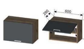
Корпус ШВГА 600 (ШхВхГ) 600x405x280 мм Фасад ШВГА 600 (ШхВхГ) 596x403x16 мм (1 шт.)
