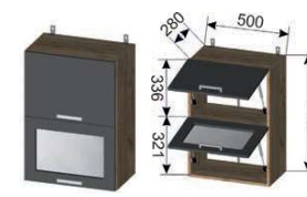
Корпус ШВГ 500 (ШхВхГ) 500x705x280 мм Фасад ШВГГС 500 (ШхВхГ) 496x350x16 мм (2 шт.)
