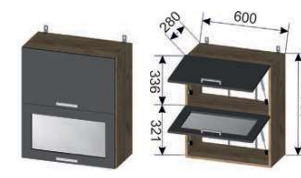
Корпус ШВГ 600 (ШхВхГ) 600x705x280 мм Фасад ШВГГС 600 (ШхВхГ) 596x350x16 мм (2 шт.)
