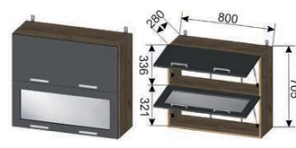
Корпус ШВГ 800 (ШхВхГ) 800x705x280 мм Фасад ШВГГС 800 (ШхВхГ) 796x350x16 мм (2 шт.)
