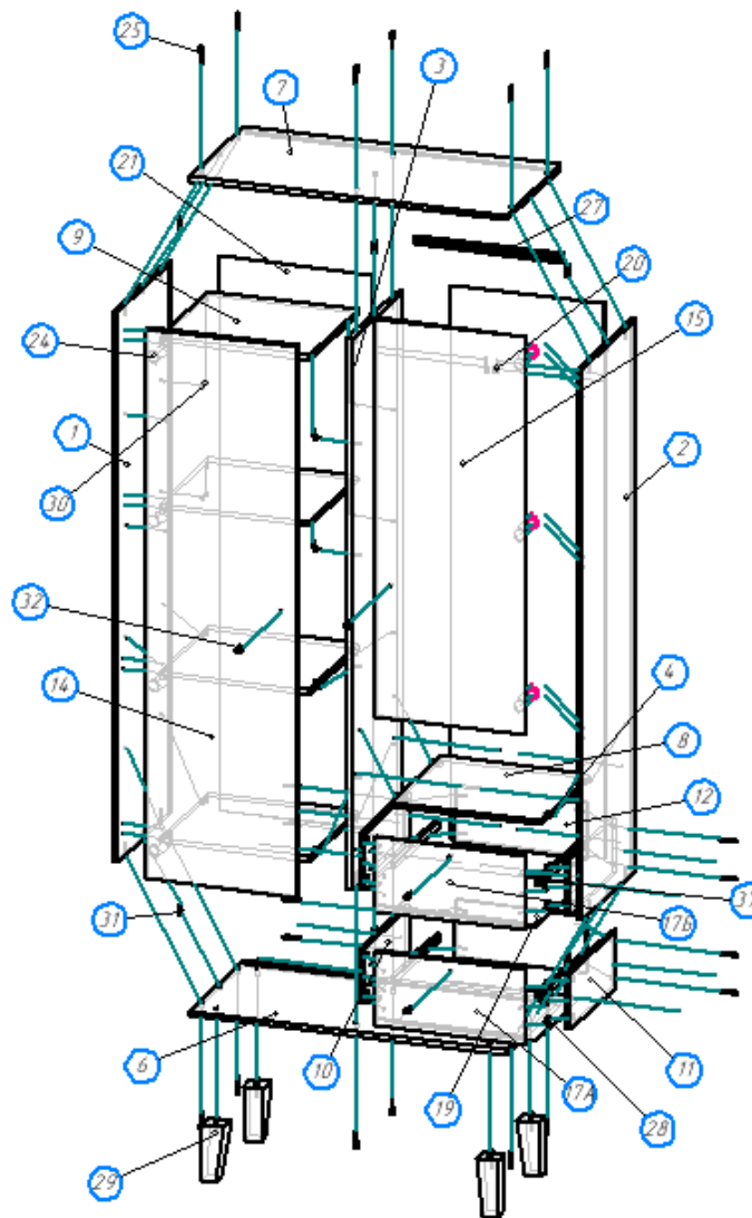
Рис.1 Сборка корпуса
