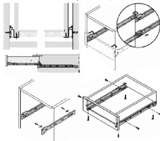
Установка направляющих ящика
