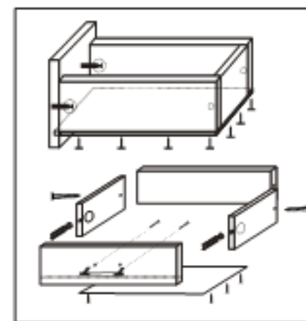
Сборка ящиков
