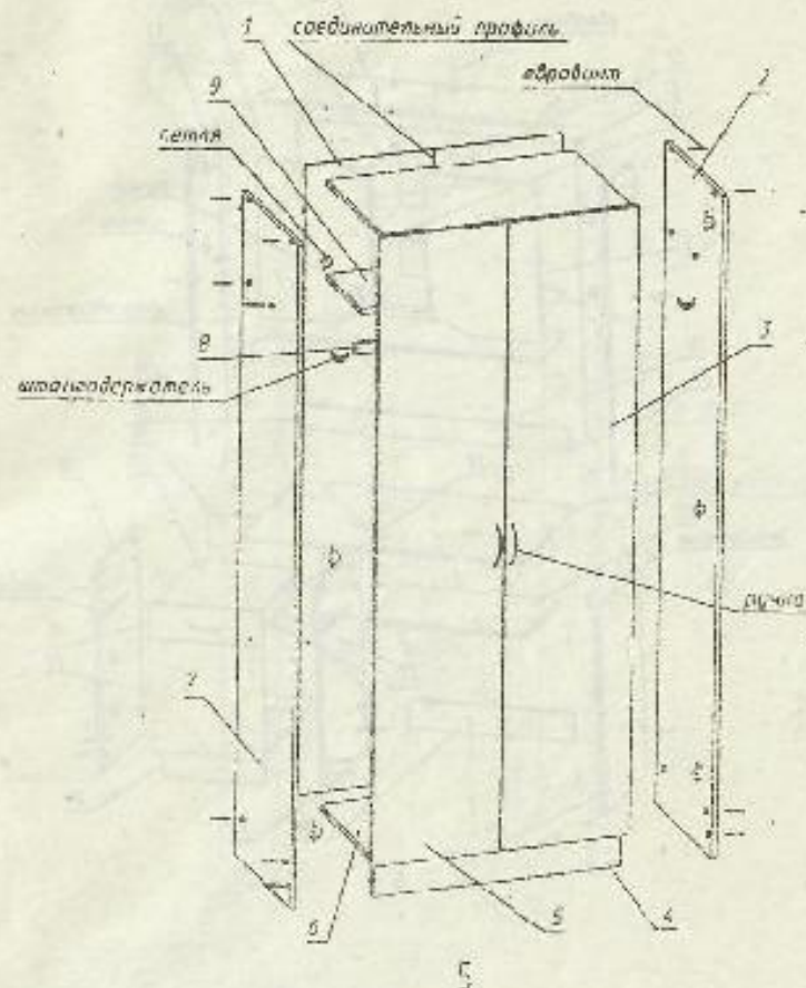
2.4. Схема сборки шкафа ШШ-01
