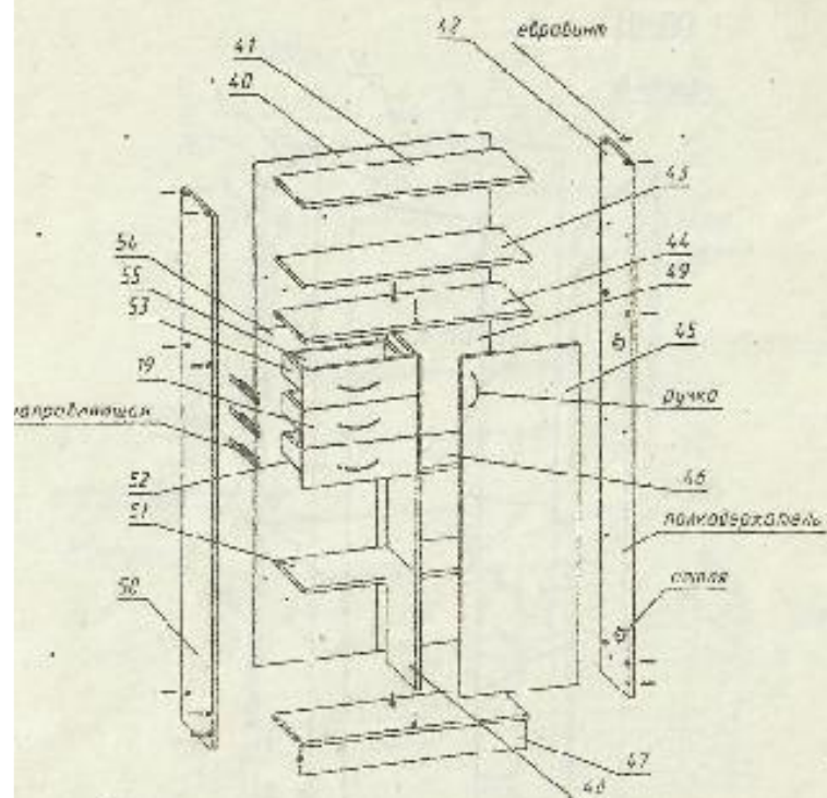
2.7 Схема сборки книжного шкафа ЮКШ-01
