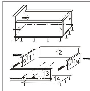
Сборка ящиков
