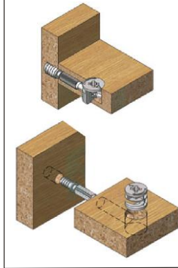
Схема сборки эксцентриковой стяжки
