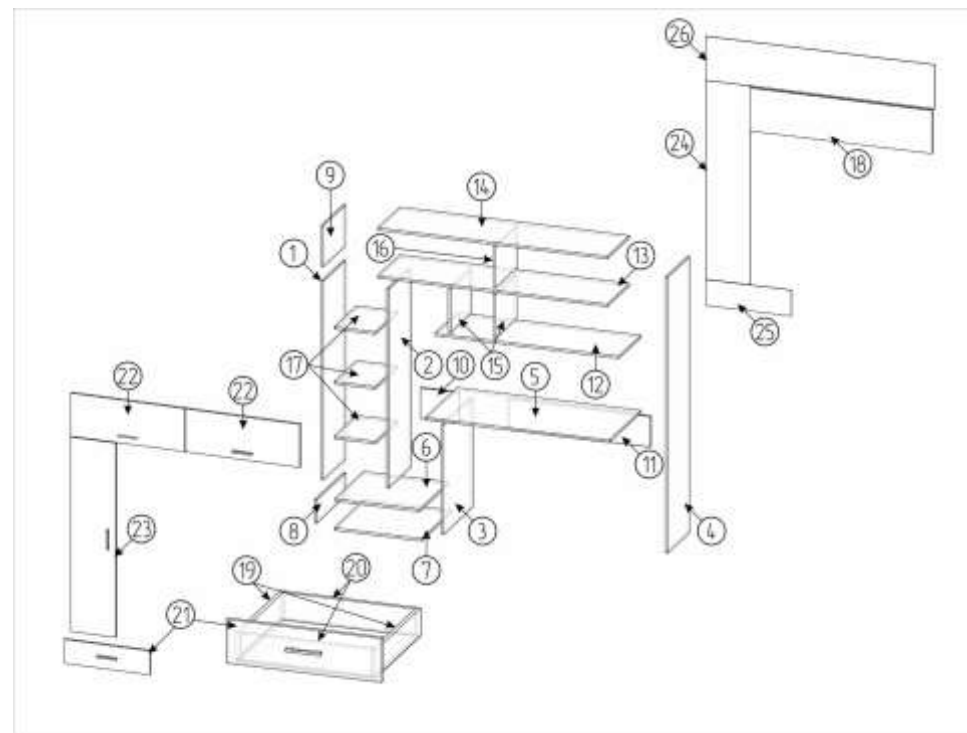
Взрыв-схема письменно-компьютерного стола ПКС-1:
