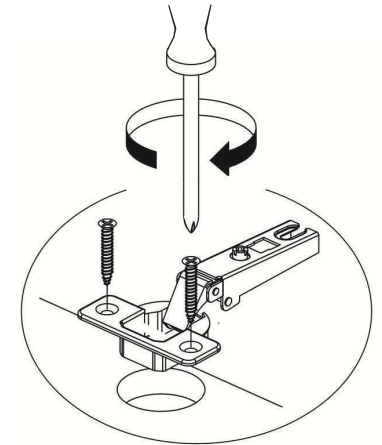
Рис.2 Монтаж чашки петли на фасад
