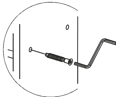
Установка евровинта
